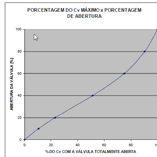
Curva do coeficiente de vazão
